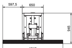
Vorderansicht
