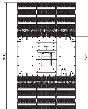
Draufsicht
