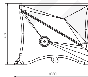
Seitenansicht
