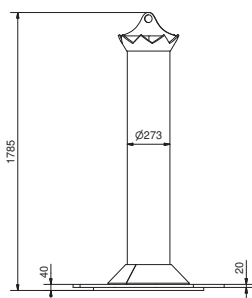
Vorderansicht
