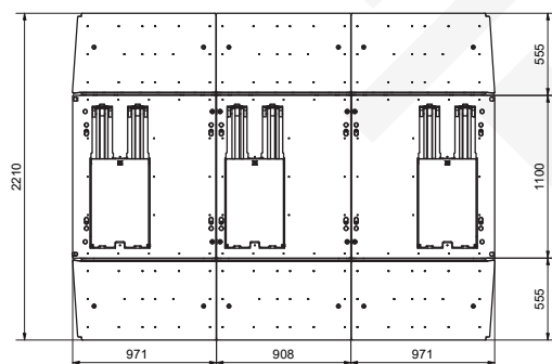
Draufsicht
