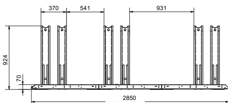
Vorderansicht
